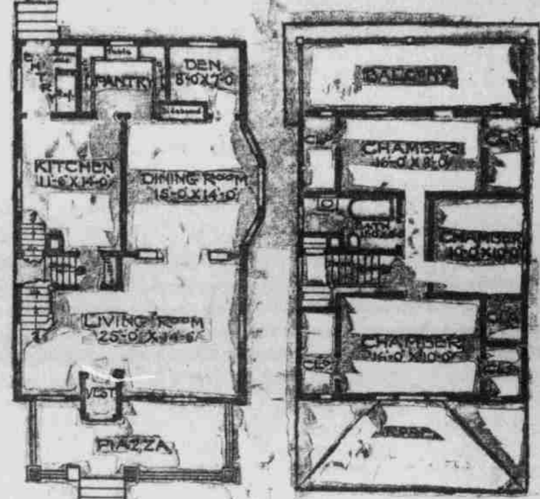
Plan des ersten Stock. Plan des zweiten Stock.
