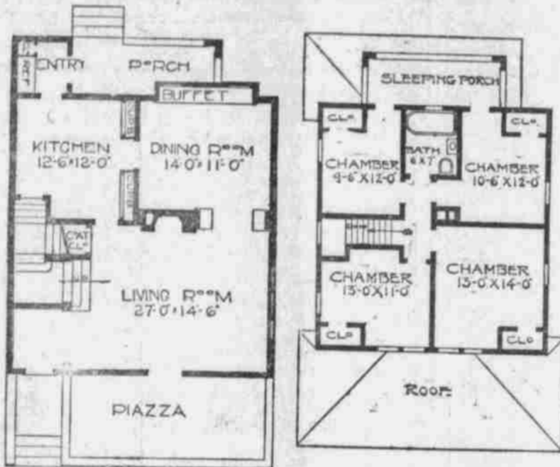
Plan des ersten Stockwerks
