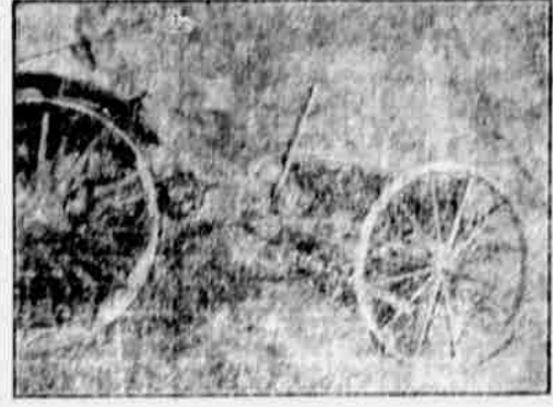
Thomas seci stroj pro traktor.
