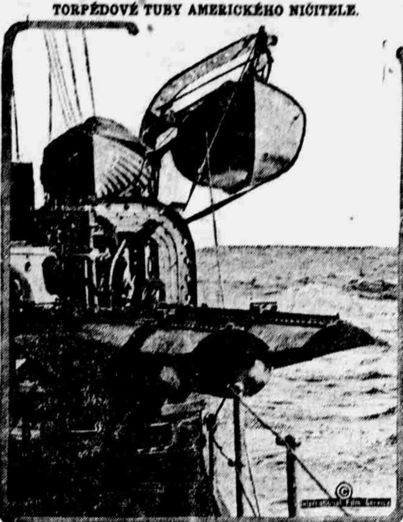
Část amerického torpédoborce, ukazující dvě torpédové tuby. Lodi těchto používá se v boji proti ponorkám.
