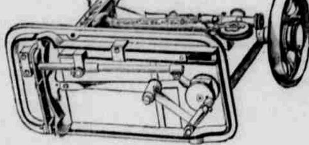
ČLUNEK jest nejnovějšího a nejjednoduššího seřízení, tak zvaný samonavíječ. Člvek vloží se do člunka, přidrží se a pohybem rotáčnímu za konec nitě jest člunek navícen.
