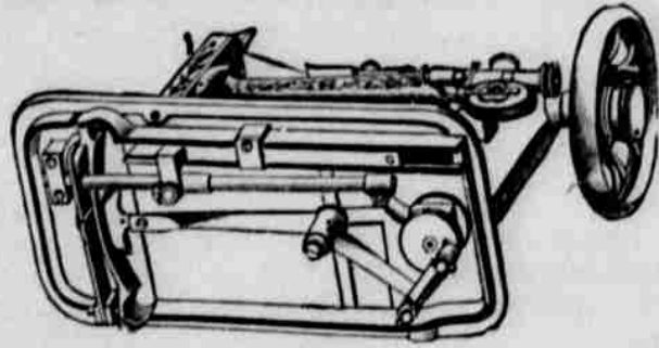
V horním vyobrazení podáváme pohled na stroj "Pokrok Západu" č. 4. Stroje tyto jsou zhotoveny ze nejdokonalejší, zručnými řemeslníky, z nejlepšího materiálu a elegantní úpravou.
