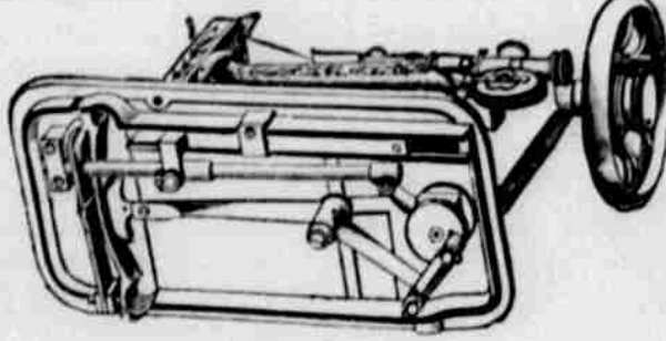
ČLUNEK jest nejnovejšího a nejjednoduššího seřízení, tak zvaný samona vláček. Cívka vloží se do člunku, přidrží se a poněkud zatáhnutím za koma nitě jest člunek navlečen.
