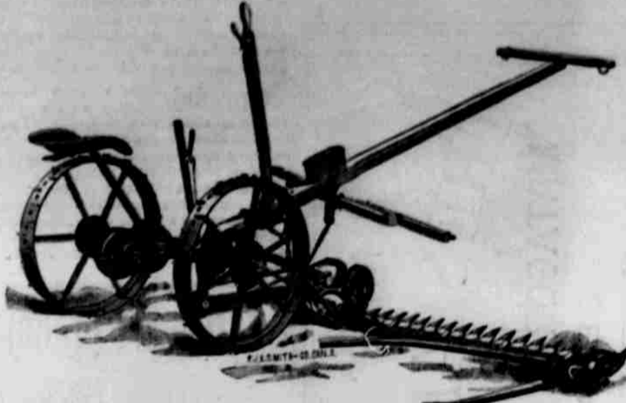
Osborne-ův sekáč č. 4. zalíží se 4, 5 a 6 stop. V lehkosti, jednoduchosti a působící sekací síle stojí v popředí před stroji jinými. Povolnost kosi činí jej spolehlivým i na nerovném povrchu, kdežto páky levé nohy a pravé ruky dostačí k úplnému Misoi jeho i hochem.
