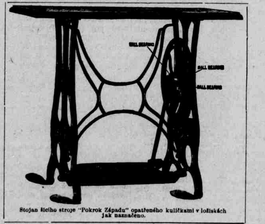
Stojan šicích strojů "Pokrok Západu" opatřených kuličkami v ložiskách...
