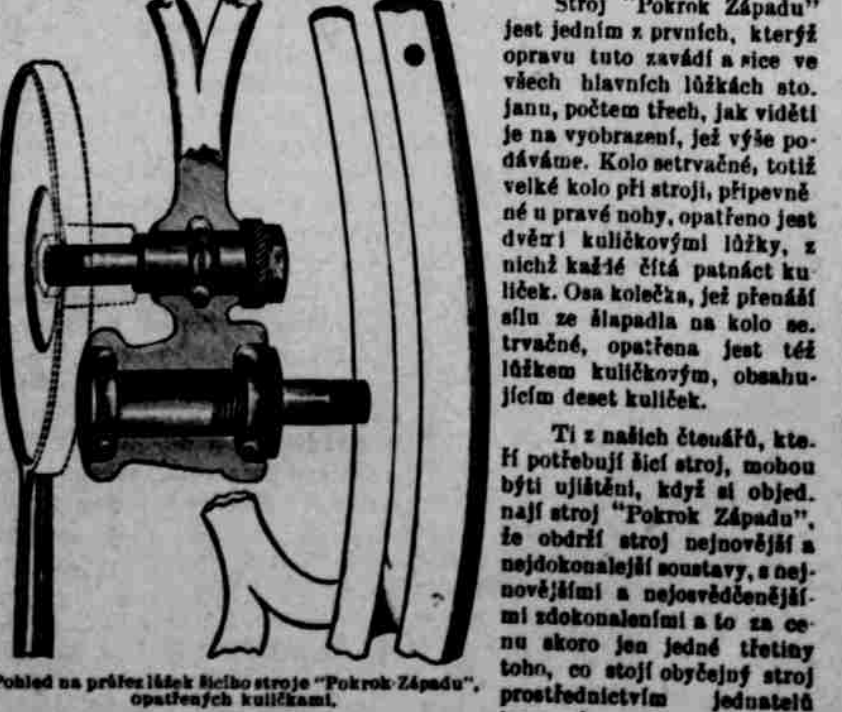
Pohled na průřez ložiska šicích strojů "Pokrok Západu" opatřených kuličkami.
