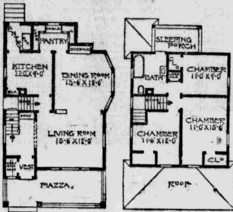
Plan des ersten Stockwerks. Plan des zweiten Stockwerks.
