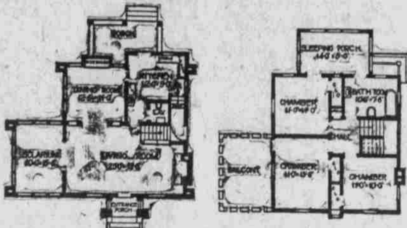
Plan des ersten Stockwerks. Plan des zweiten Stockwerks.
