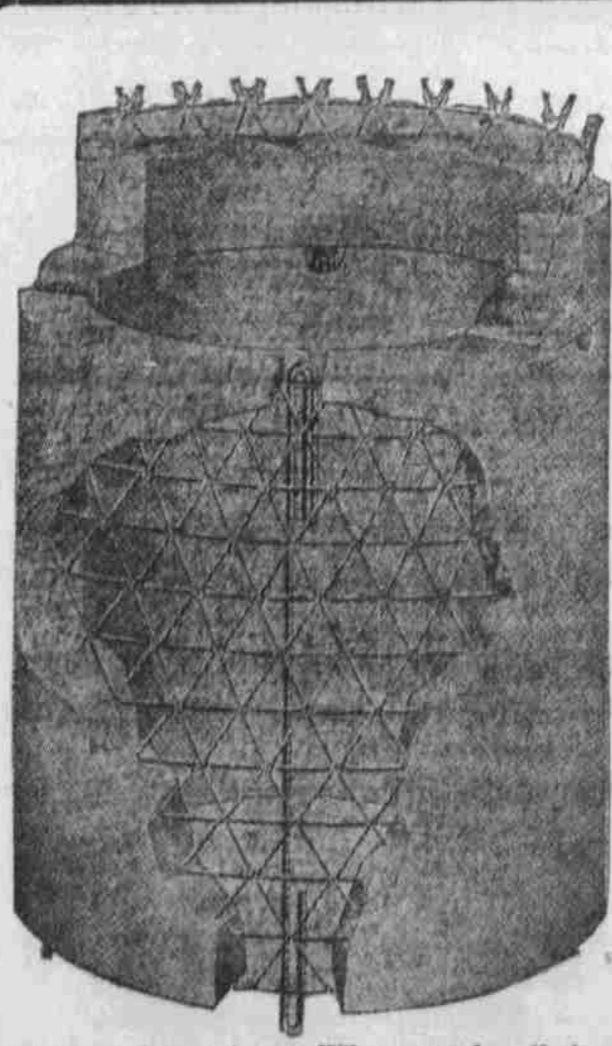
Die Konstruktionsweise von Wilson verstärkten Konkret-röhren für Silos, Culverts, Abflusströhren und vieles andere
