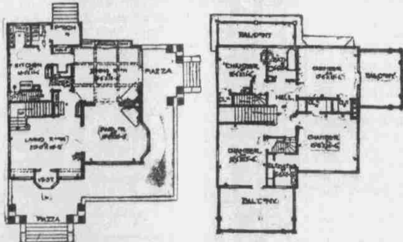
Plan des ersten Stocks
