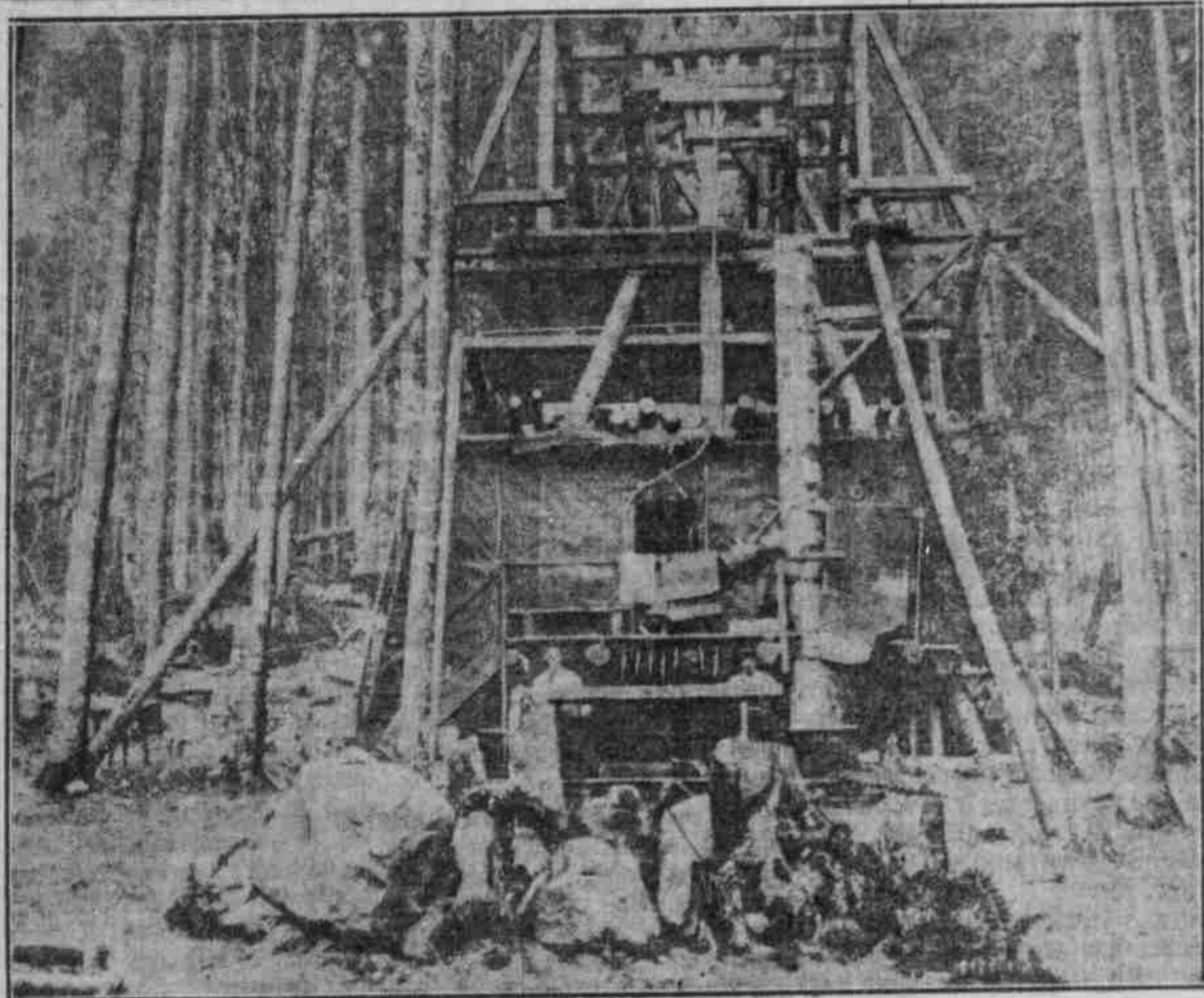
Schwebefahrbahn am Hartmannsweilerlopf, von unten gesehen.
