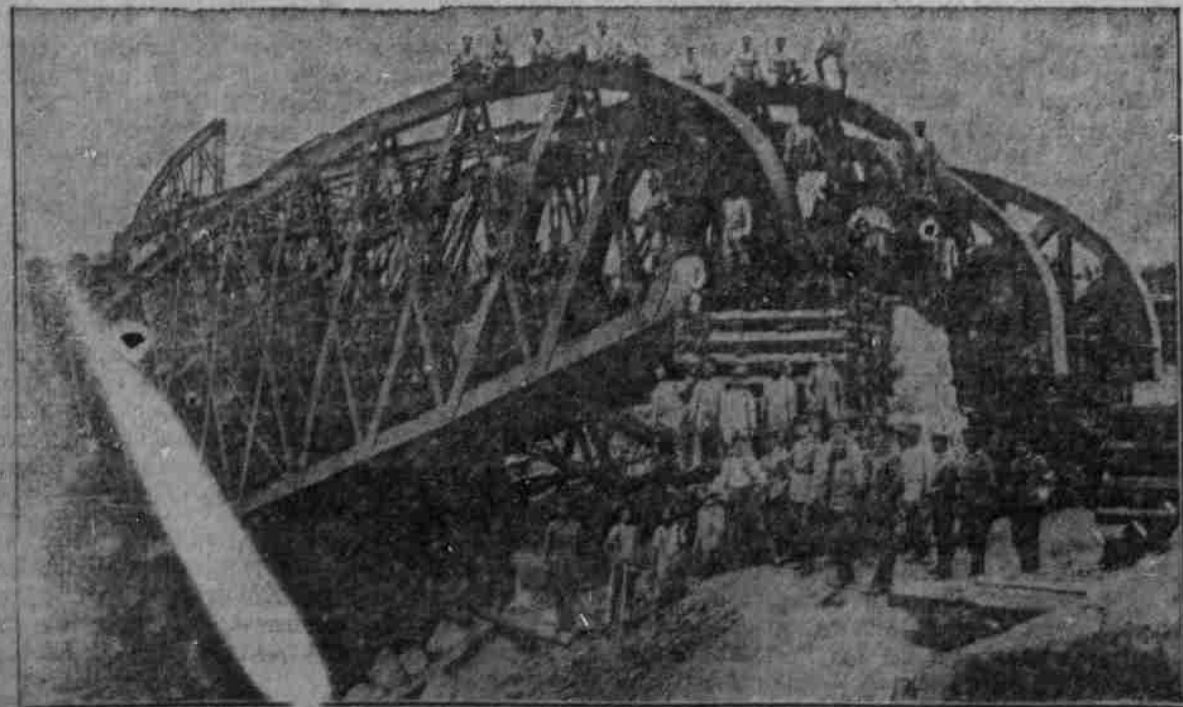
Eine von den Russen gesprengte Eisenbahnbrücke bei Lemberg wird von Berliner Eisenbahnerkomp. wieder aufgebaut.
