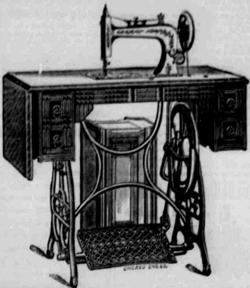
V horním vyobrazení podáváme pohled na stroj "Pokrok Západu" č. 4. Stroj tyto jsou zhotoveny co nejdokladněji, zručnými řemeslníky, z nejlepšího materiálu a elegantní úpravy.
