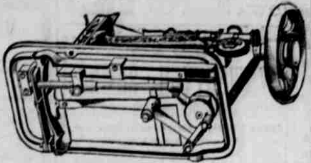
V horním vyobrazení podáváme pohled na stroj "Pokrok Západu" č. 4. Stroj tyto jsou zhotoveny co nejdokladněji, zručnými řemeslníky, z nejlepšího materiálu a elegantní úpravy.
