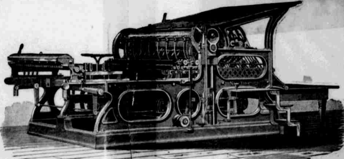
VYTVARAČNÍ STROJE POTTEROVA.
